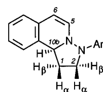
33a Ar = C 6 H 5 34b Ar = C 5 H 4 N-(2)
